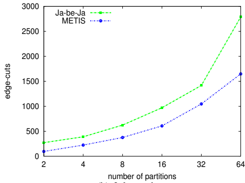
(b) 3elt graph.
